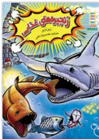
زنجیره‌های غذایی
