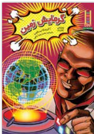
گرمايش زمين
