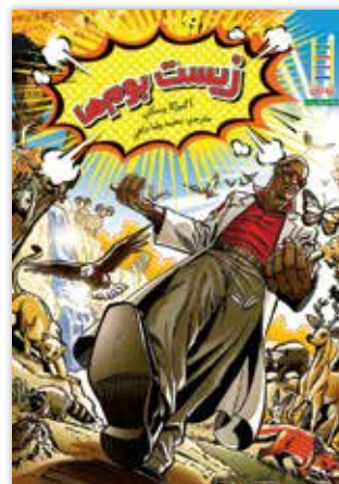
زیست بوم‌ها
